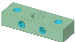
Art: 15054 Underlägg 150x50x32 Med ett fästhål samt tvärgående M16
