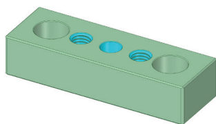
Art: 15050 Underlägg 150x50x32 Med två fästhål
